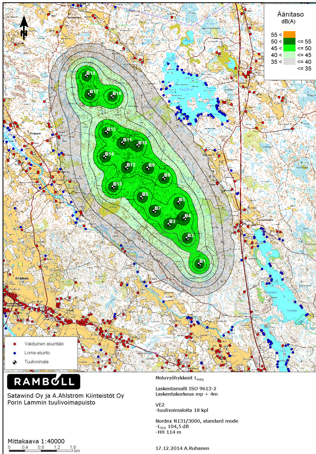
Kuva 17-2. Melumallinnus vaihtoehdossa 2.
