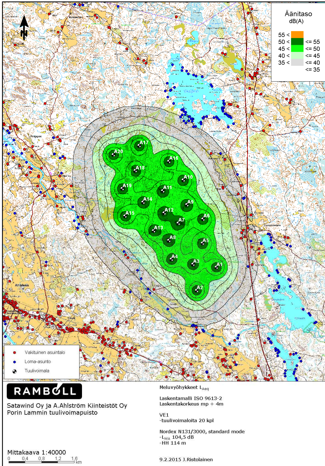
Kuva 17-1. Melumallinnus vaihtoehdossa 1
