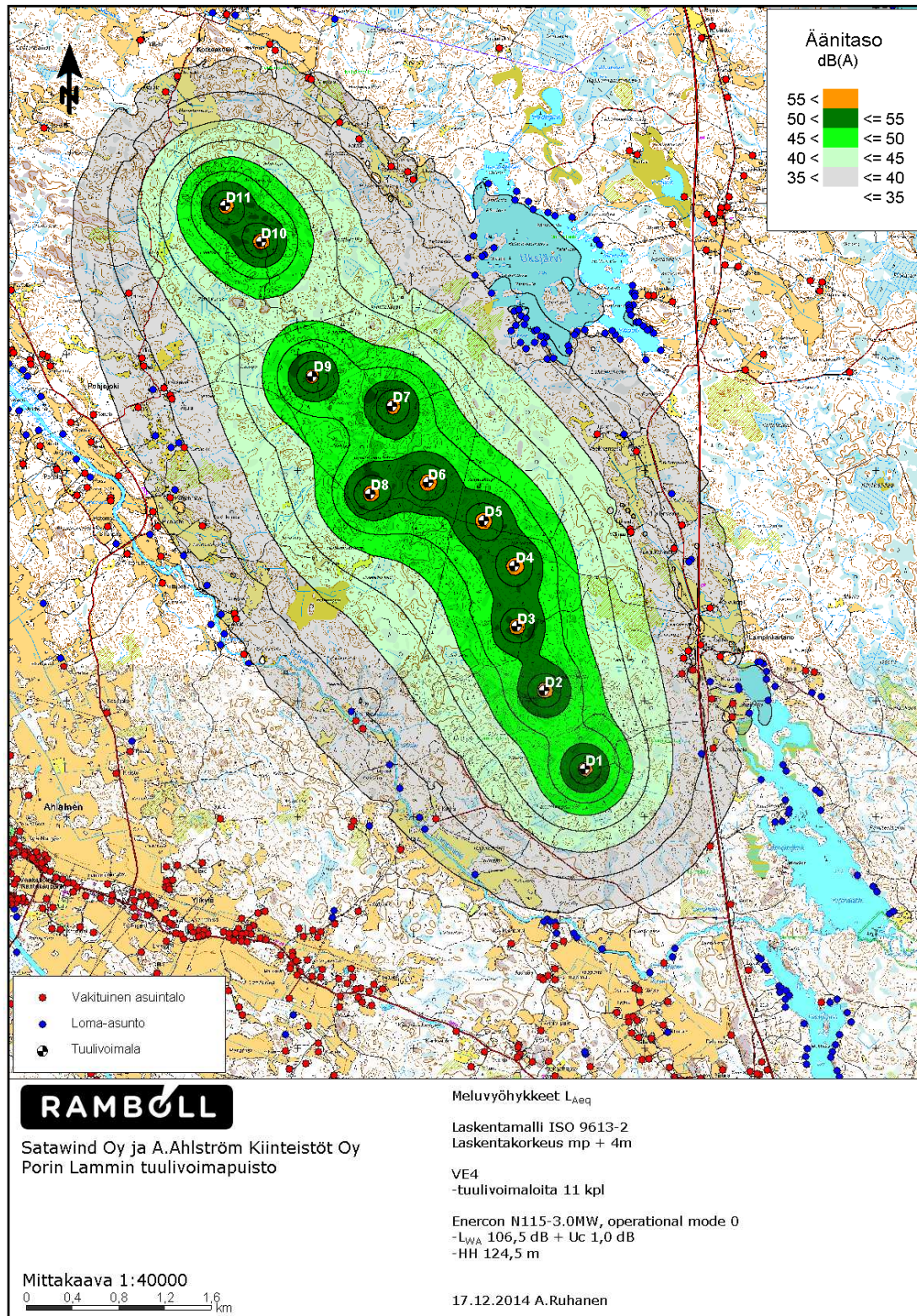
Kuva 17-4. Melumallinnus vaihtoehdossa 4.
